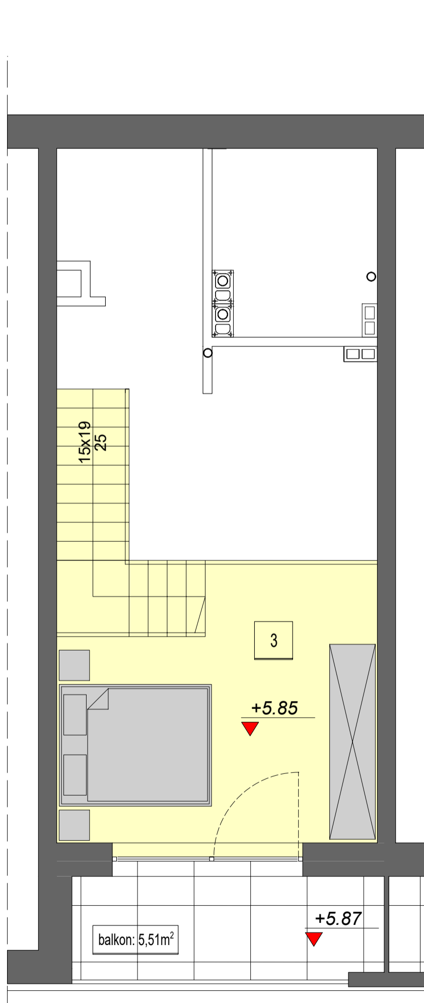
RZUT ANTRESOLI
