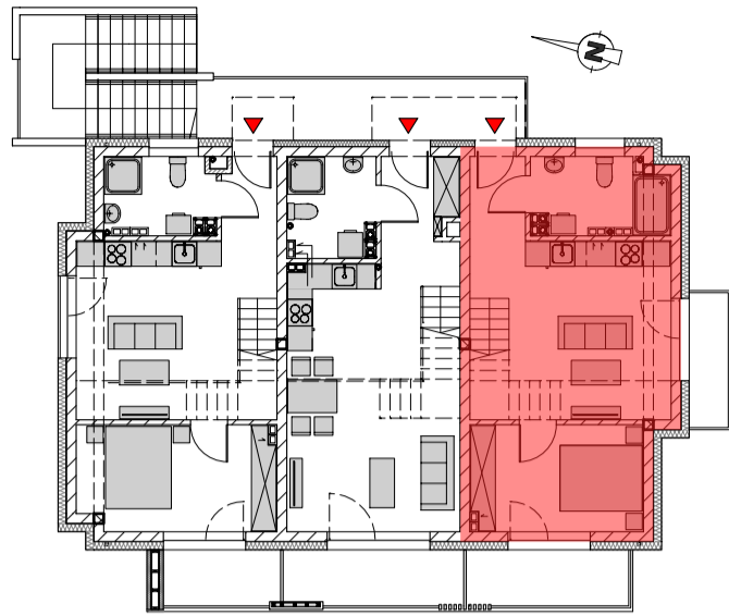
RZUT ANTRESOLI
