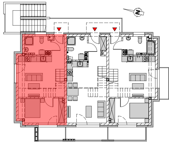
RZUT ANTRESOLI
