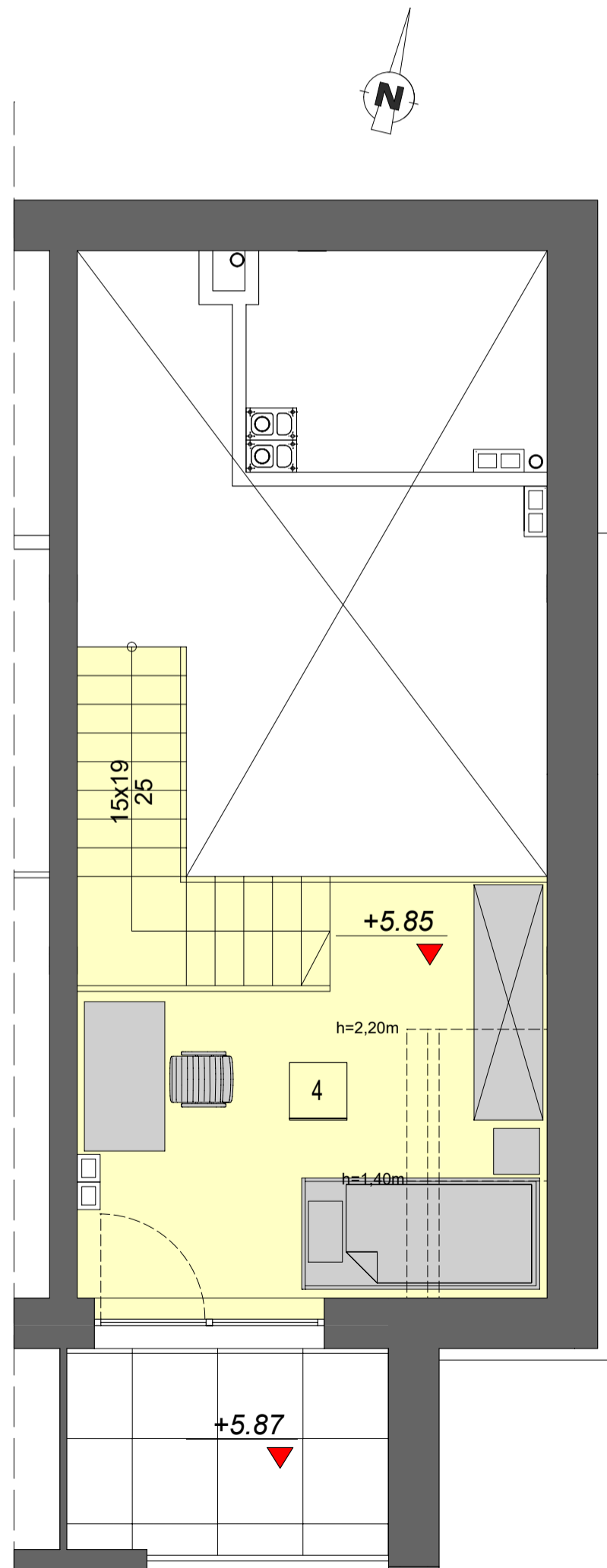
RZUT ANTRESOLI
