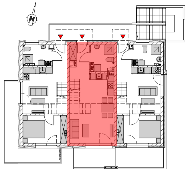
RZUT ANTRESOLI
