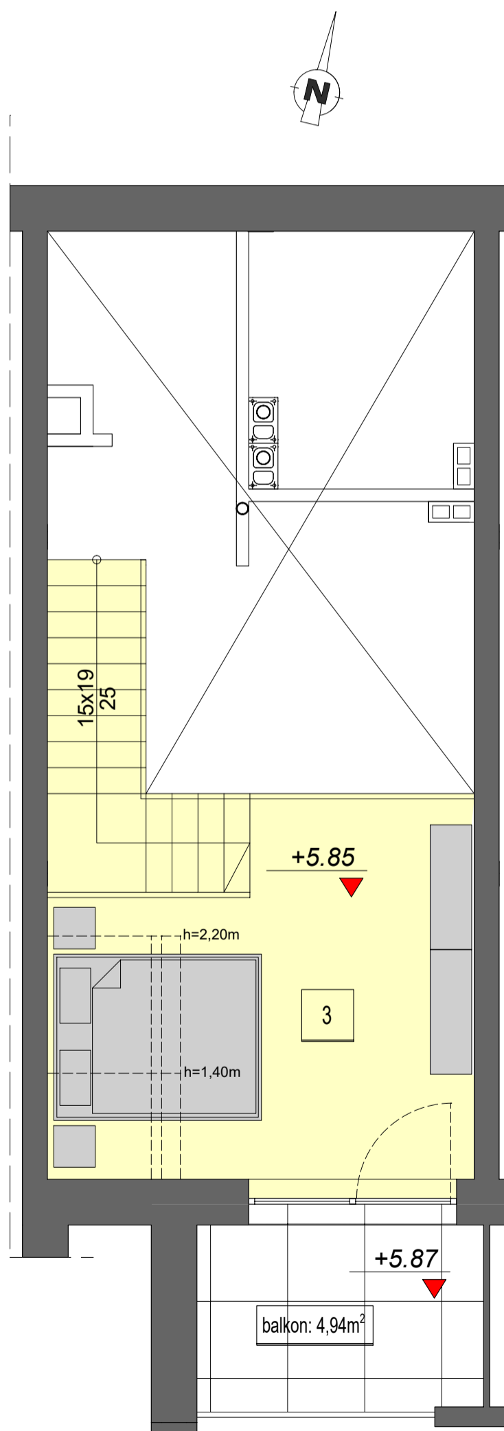
RZUT ANTRESOLI
