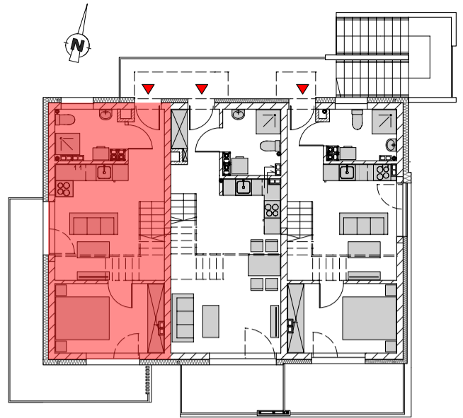
RZUT ANTRESOLI
